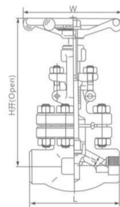
焊接阀盖示意图 Welded bonnet
