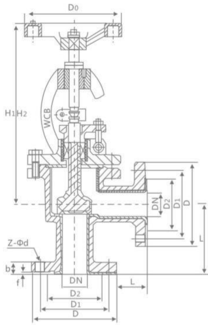
J44 F46 F3 型法兰连接手动截止阀(角式)
